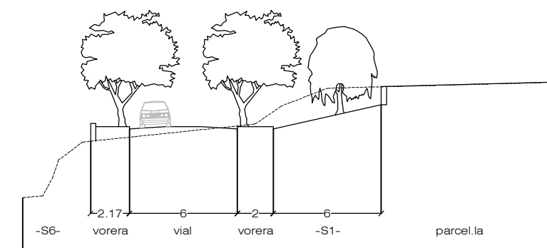
secció 2 escala= 1:300
