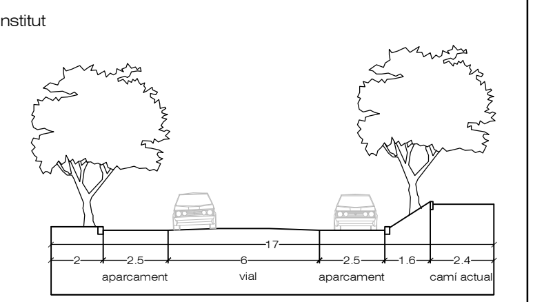
secció 1 escala= 1:200
